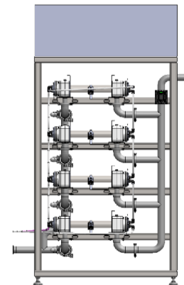
大流量タイプ ≤1,400L/Min
