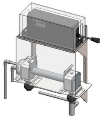
中流量タイプ ≤100L/Min
